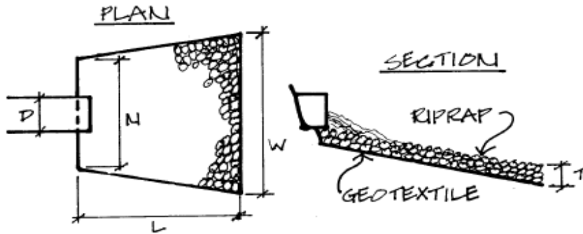
Rock Apron
